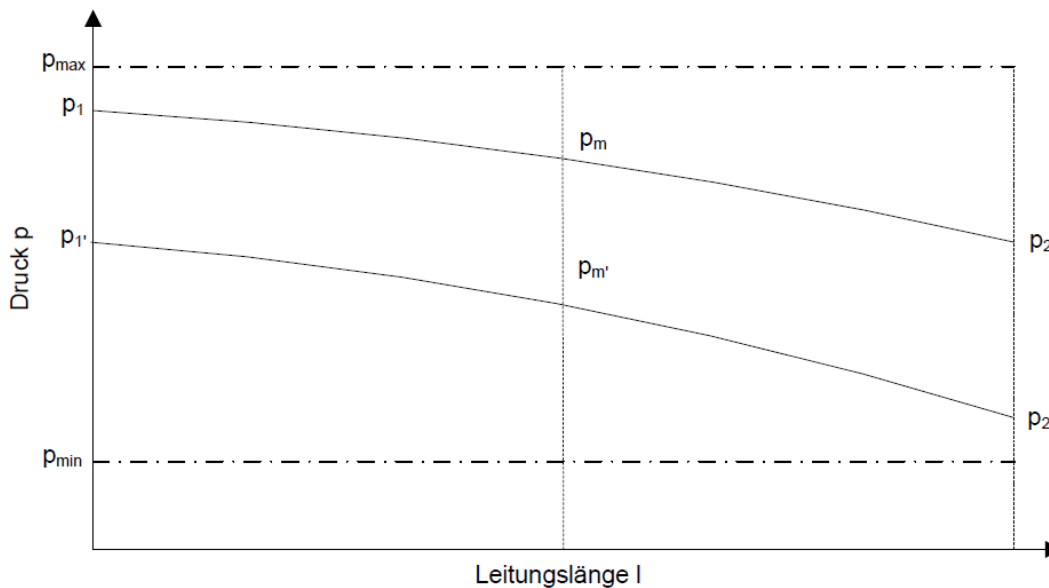
Bild 1 – Druckverläufe in einer geraden Leitung.
